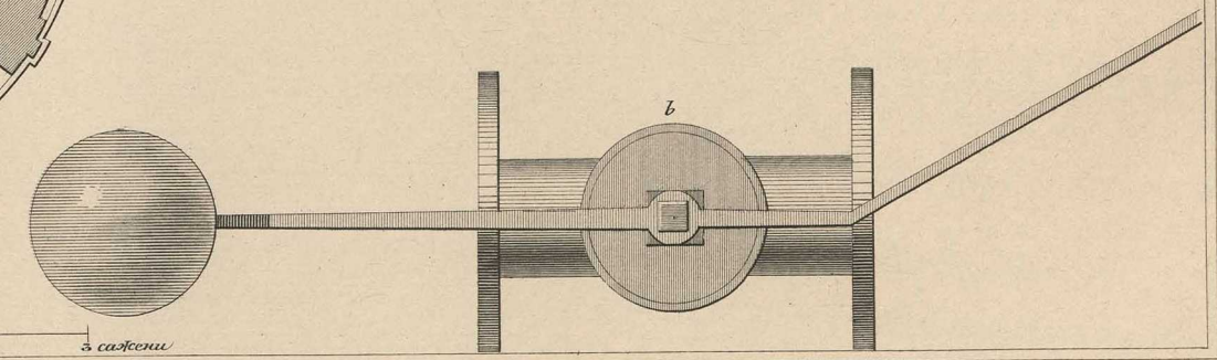
Мааситабъ къ чертежу А.В.В.Г.
